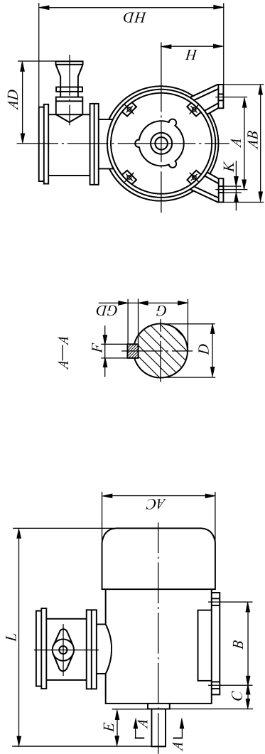
图 A.1 泵用隔爆型三相异步电动机外形结构图
