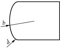
b —冲头半径,(30±0.15)mm; d —转角半径,0.80 mm。
