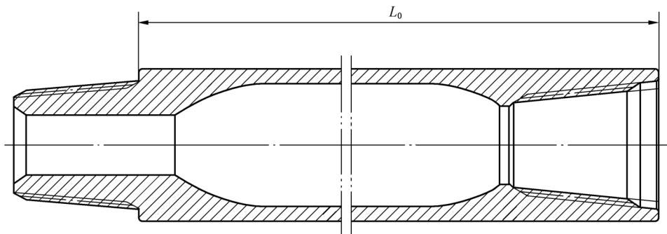
图 1 整体型钻杆
