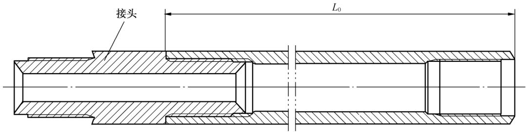
图 2 接头联接型钻杆
