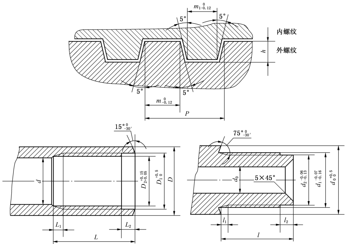
图 4 接头联接型钻杆及接头螺纹牙型
