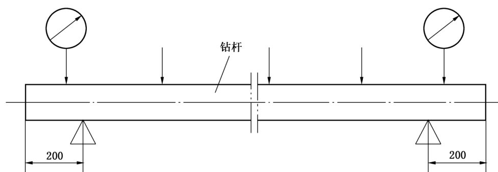
图 5 钻杆直线度测量
