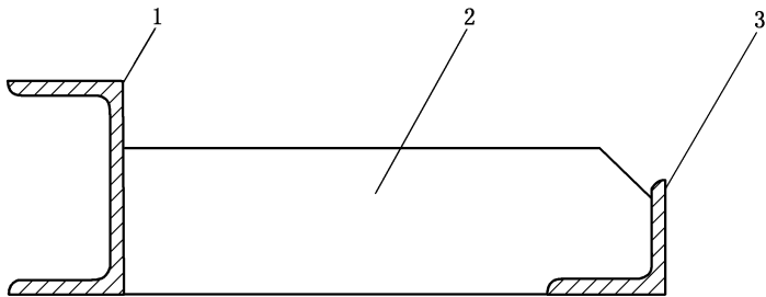
图 2 单钢板法兰盘截面
