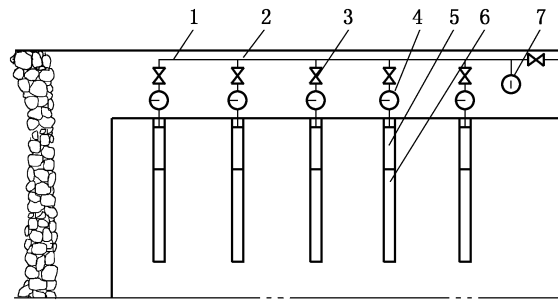
1—钢丝编织高压胶管;2—接头;3—阀门;4—注水表; 5—封孔器;6—注水管;7—压力表
