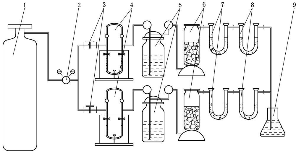
1—钢瓶；2—减压器；3—流量调节器；4—毛细管流量计(内装液体石蜡)；5—洗气瓶； 6—干燥塔；7—U形带支吸收管(前半部盛装氢氧化钙试样,后半部盛装用二氧化碳 饱和过的无水氯化钙)；8—U形带支吸收管(内装无水氯化钙)；9—三角瓶。
