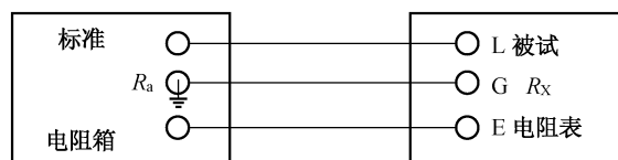
图 1 绝缘电阻表误差试验接线图
