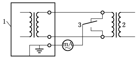
1—可触及导电件;2—电网电压;3—转换开关
