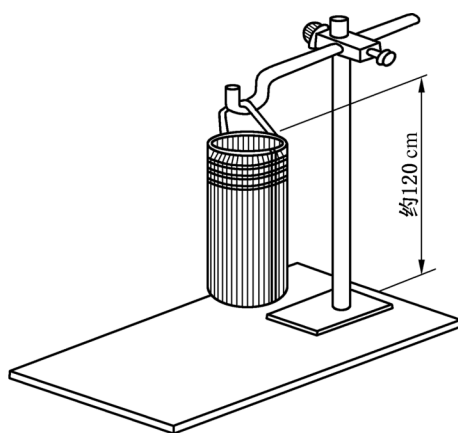
图 B. 2 发烟试验台
