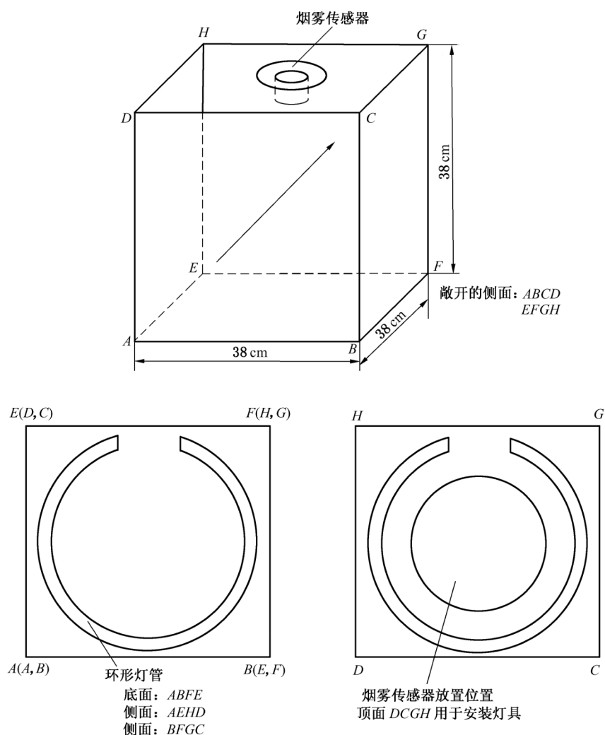
图 A.1 闪光装置
