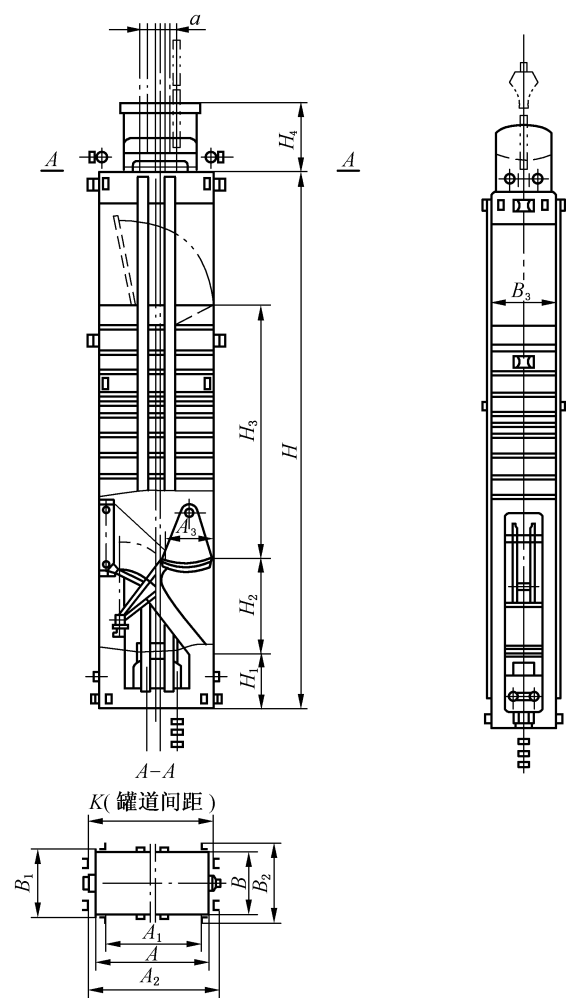
图 3 32,40,50t 同侧装卸式箕斗
