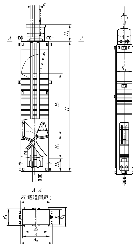
图 4 32,40,50t 异侧装卸式箕斗
