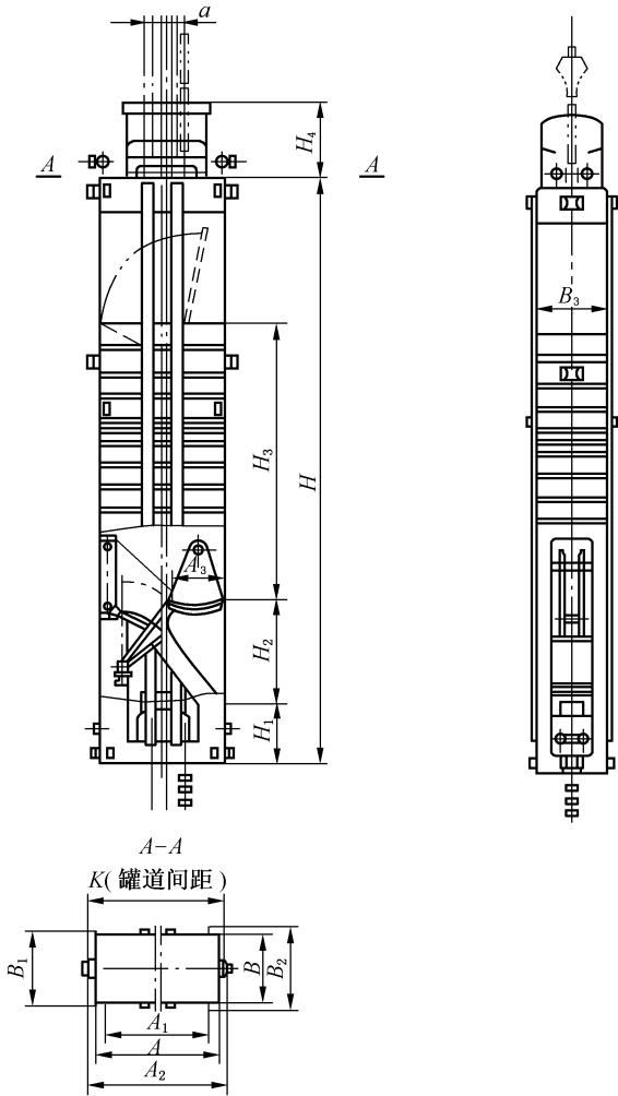
图 2 20,25t 异侧装卸式箕斗
