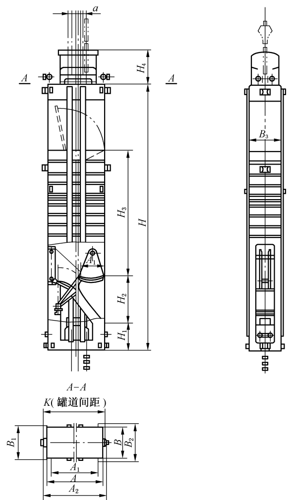
图 1 20.25t 同侧装卸式箕斗
