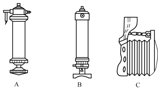
A—圆筒形抽入式;B—圆筒形真空式;C—蛇腹形
