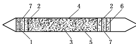
1—起始端衬塞;2—隔离层;3—指示粉;4—分度线;5—玻璃管;6—衬塞;7—保护层
