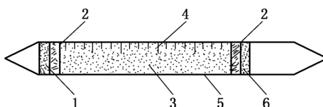
1—起始端衬塞;2—隔离层;3—指示粉;4—分度线;5—玻璃管;6—衬塞
