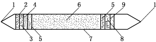
1—管尖;2—起始端衬塞;3—除水层;4—除干扰层;5—隔离层; 6—指示粉;7—玻璃管;8—保护层;9—衬塞
