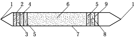
1—管尖;2一起始端衬塞;3—除水层;4—除干扰层;5—隔离层; 6—指示粉;7—玻璃管;8—保护层;9—衬塞
