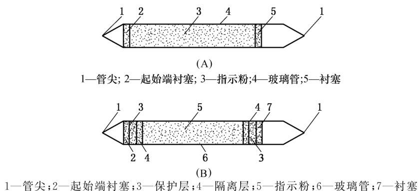
图 1 二氧化硫检测管示意图
