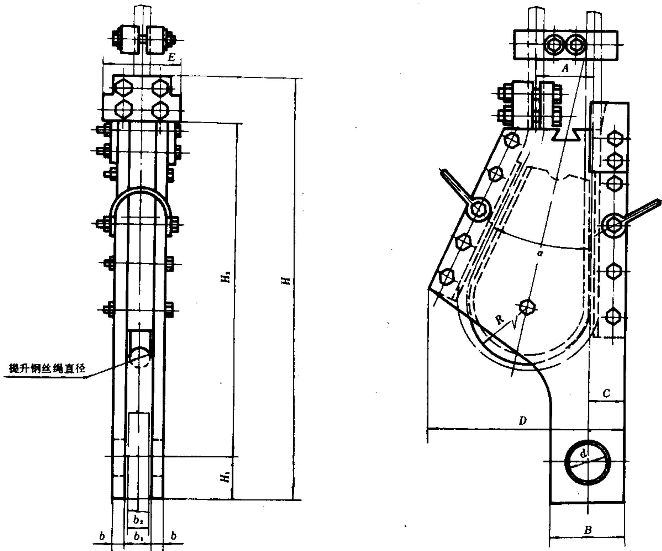
楔形绳卡图
