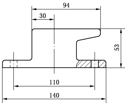
图2 导轨衬Ⅱ型(平形)
