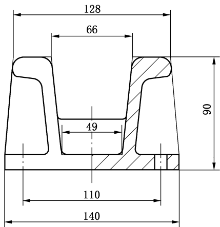
图1 导轨衬Ⅰ型(槽形)
