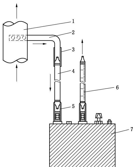
1—柴油机排气管；2—取样探头；3、5—取样管；4—CO 除干扰管或 \text{NO} \rightarrow \text{NO}_2 氧化管； 6—CO 或 \text{NO}_2 检测管；7—电子气体自动采样器
