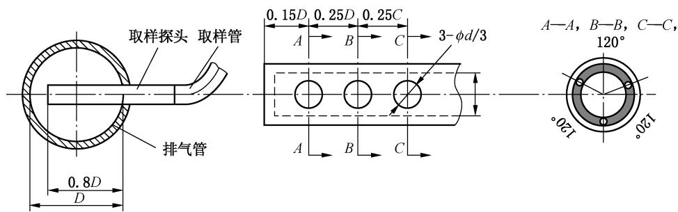
图 B1 推荐的取样探头示意图
