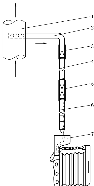
1—柴油机排气管；2—取样探头；3、5—取样管；4—CO 除干扰管或 \text{NO} \rightarrow \text{NO}_2 氧化管； 6—CO 或 \text{NO}_2 检测管；7—负压吸入式采样器
