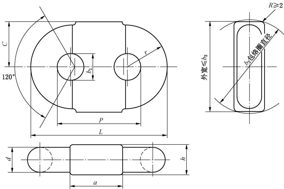
图 1 扁平接链环
