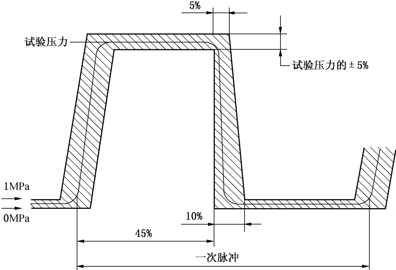
图 3 脉冲压力波形
