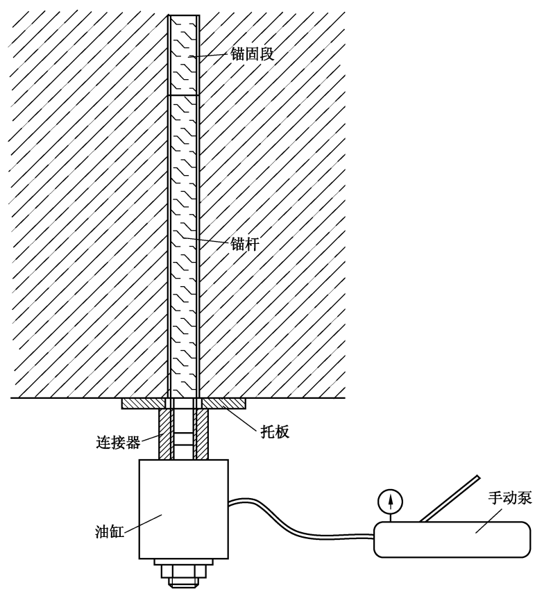
图 A.1 锚杆拉拔力试验示意图
