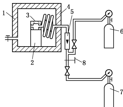
1—试验箱;2—仪器;3—注气装置;4—预热盘管;5—流量计; 6—清洁空气瓶;7—试验气样瓶;8—调节阀
