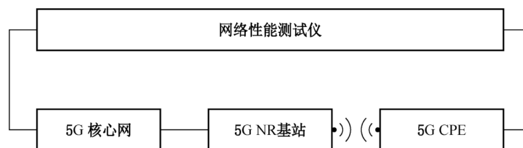
图 2 SA 组网架构示意图
