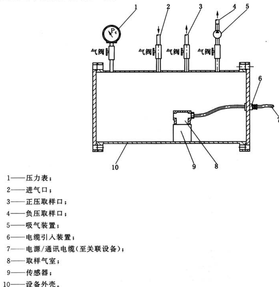
图 1 压力影响试验装置结构示意图
