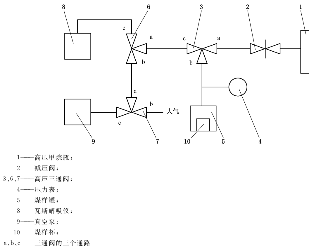
图 1 测定钻屑瓦斯解吸指标实验系统示意图
