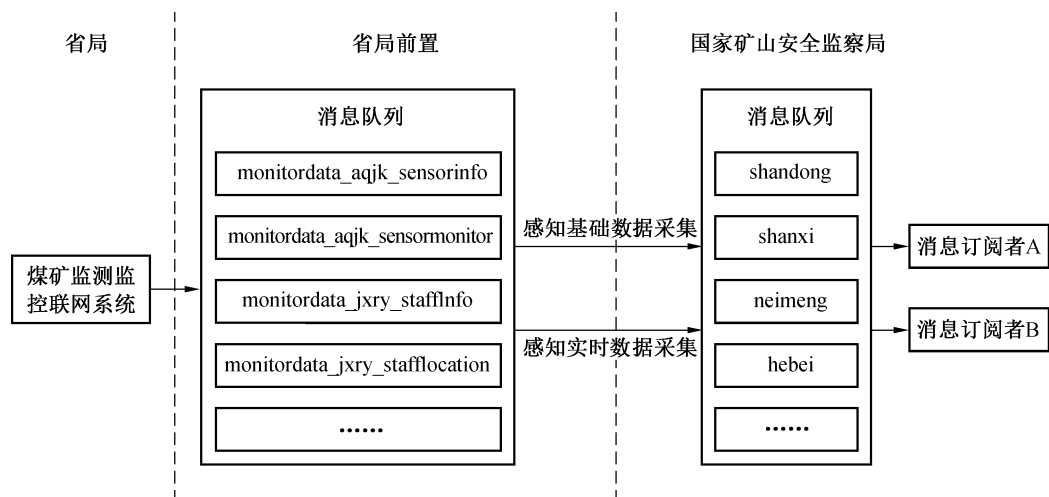
图 2 消息队列对接方法示意图
