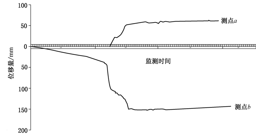
(a) 测点位移历时曲线
