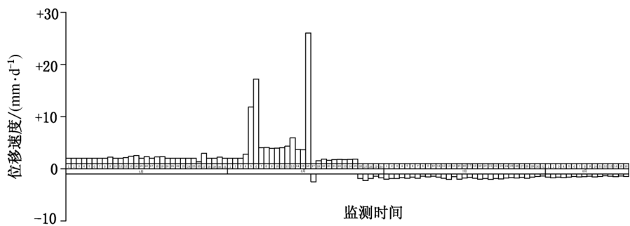
(b) 测点位移速度历时变化曲线
