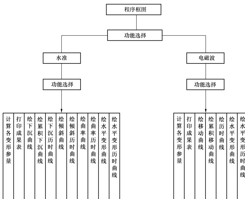
图 3 地表位移监测数据分析程序框图
