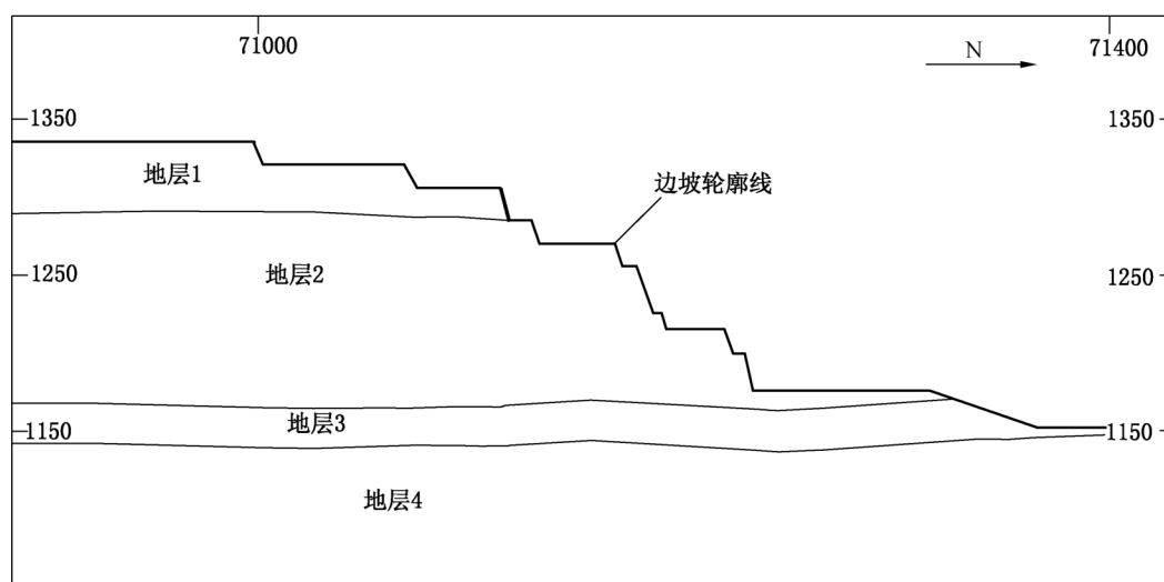
图 D. 1 地质剖面图
