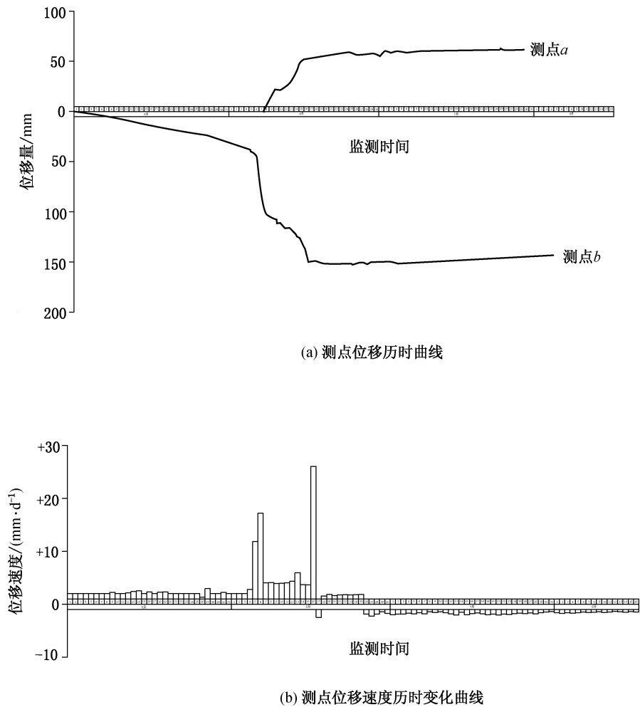
图 I. 1 边坡岩体地表位移监测成果曲线
